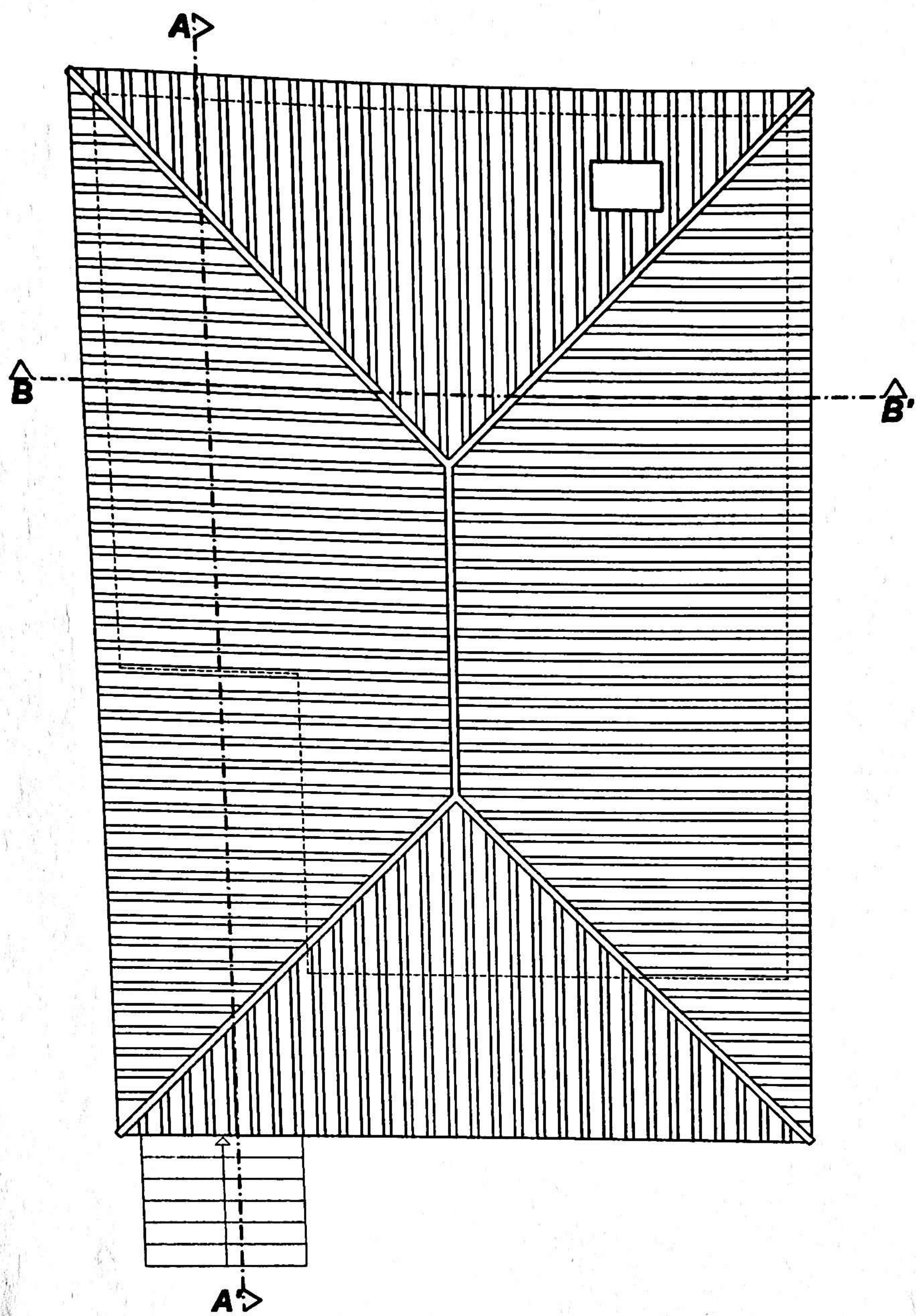
PLANTA DA COBERTURA
