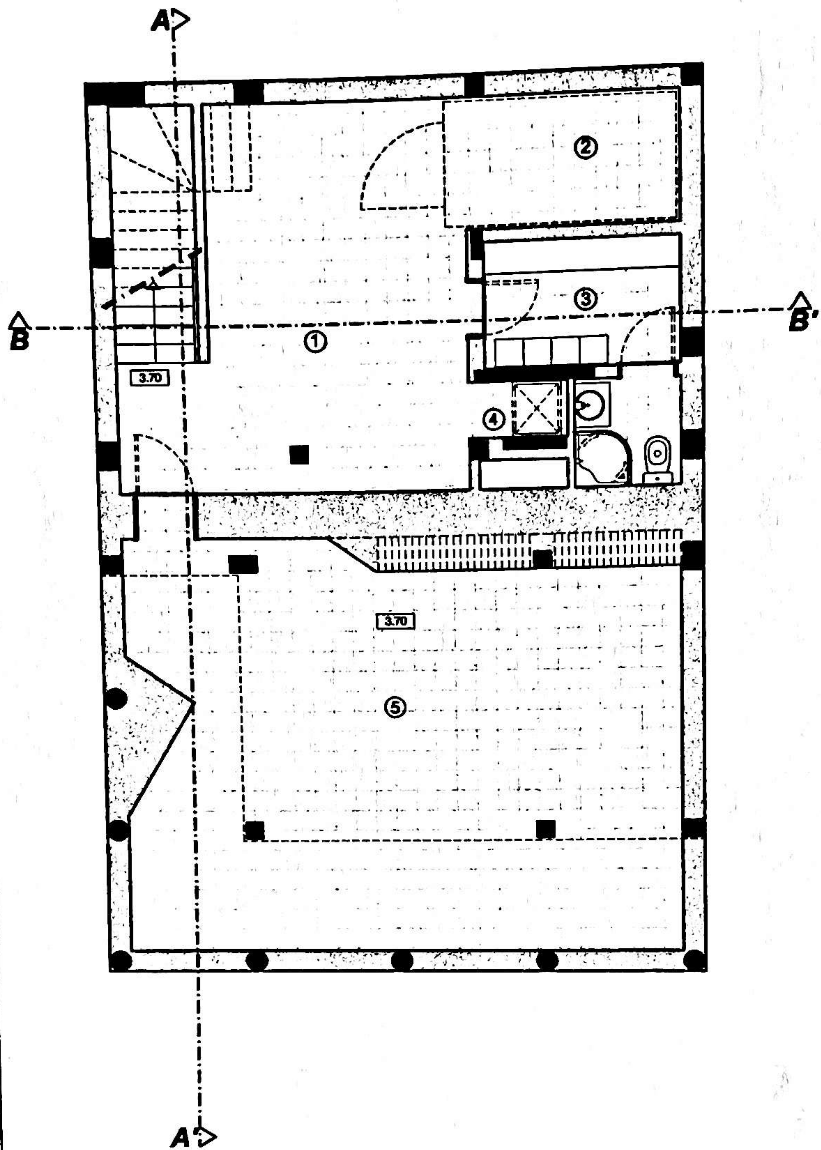
PLANTA DA CAVE
