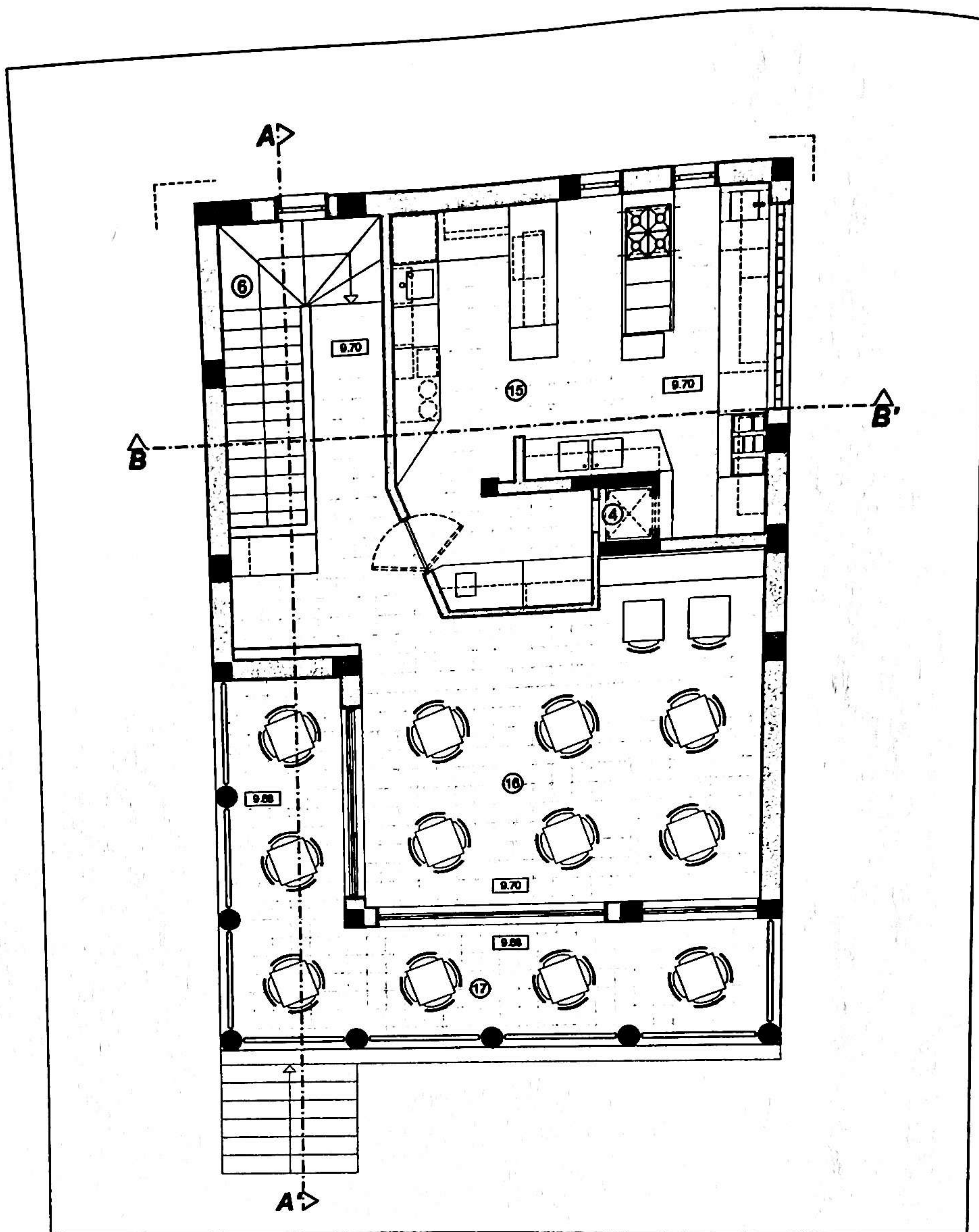
PLANTA DO 1º ANDAR
